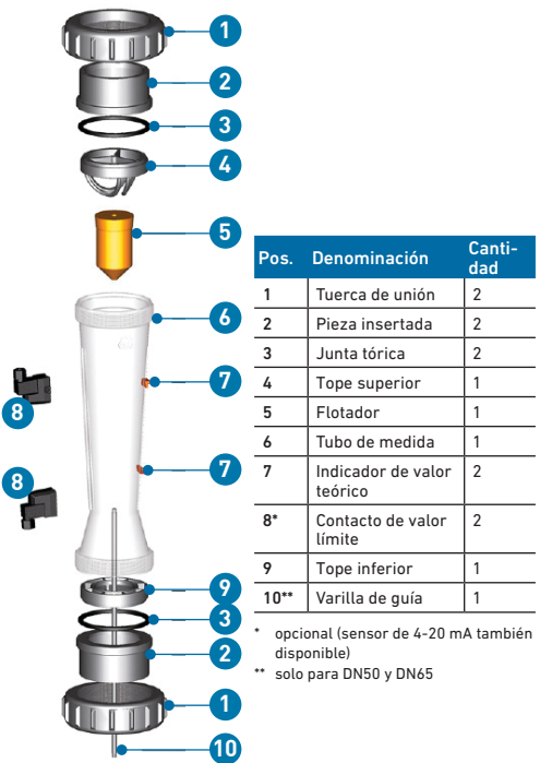
Fig. 1: Caudalímetro de área variable
