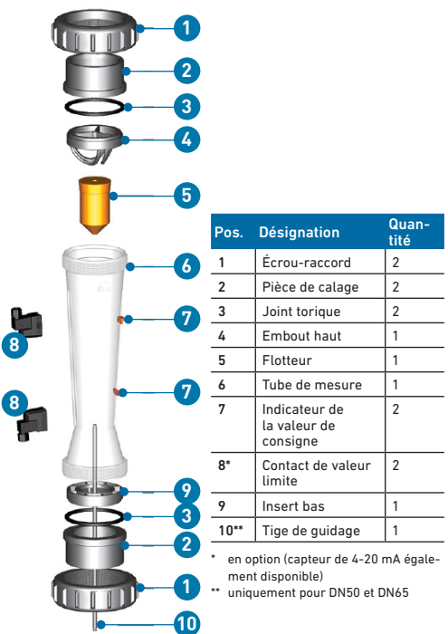
Fig. 1 : Débitmètre avec flotteur
